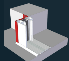
C: Montageprofil hinter der lichten Breite
