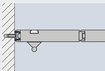
Schiebetor ohne Einlaufprofi
