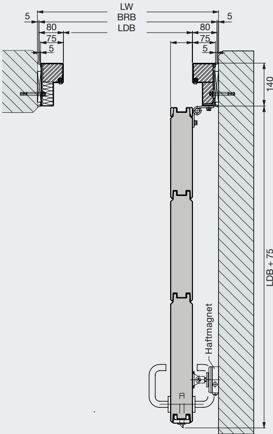
90° Offenstellung
