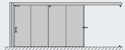
Teleskop-Schiebetor
