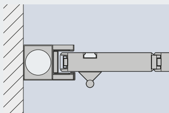
Schiebetor mit Einlaufprofi
